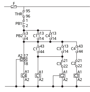
Bağlantı Şeması 2 (HGC115 ~ 800)
