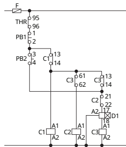
Bağlantı Şeması 1 (HGC9 ~ 100)
