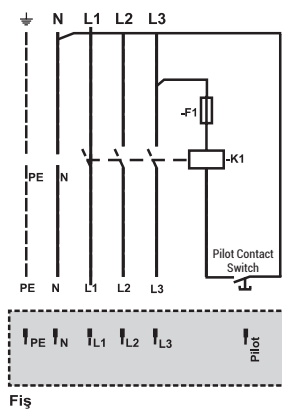
Pilot Kilit Mekanizması
