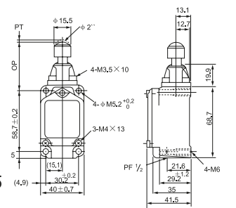
CWLD3 TGB-5-111 Pimli Siviç Kutu/Koli : 10/80 Fiyat : $32,75
