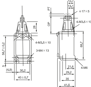
CWLD1 TGB-5-110 Makaralı Siviç Kutu/Koli : 10/80 Fiyat : $32,75
