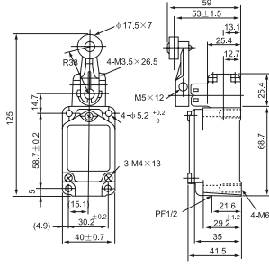
CWLCA2-2 TGB-5-104 Yatay Kol Makaralı Kutu/Koli : 10/90 Fiyat : $32,75
