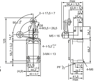
CWLCA32-41 TGB-5-105 Yön Sivici Kalıcı Kutu/Koli : 10/80 Fiyat : $32,75
