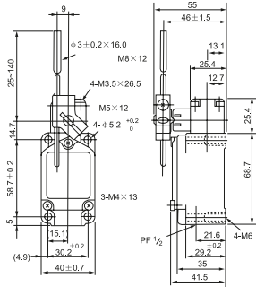
CWLCL TGB-5-107 Ayarlı Çubuk Kutu/Koli : 10/90 Fiyat : $32,75
