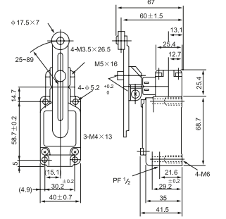
CWLCA12-2-Q TGB-5-108 Açısal Ayarlı Kol Kutu/Koli : 10/90 Fiyat : $32,75
