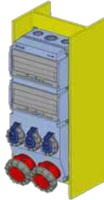
L Profil Çelik Konstrüksiyon Arasına Kolay Montaj
