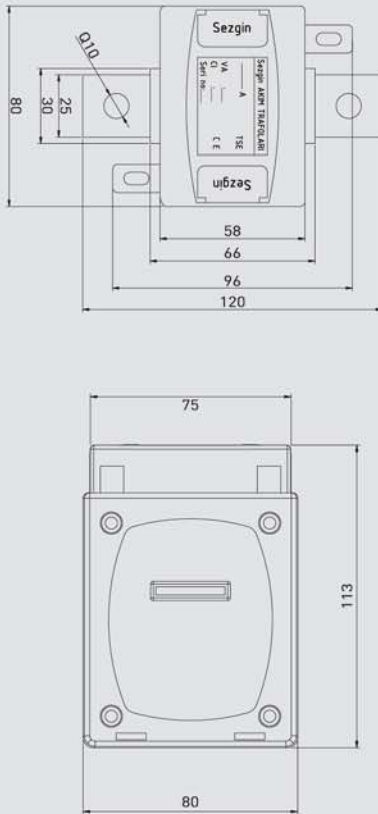
Teknik Resim
