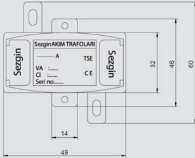
Teknik Resim
