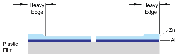
Dayanıklı Kenar Metalizasyon Film İç Yapısı
